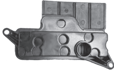
AISIN WARNER U660E, U660F Pan Gasket U660E.GAS01 Filter U660E.FIL01
