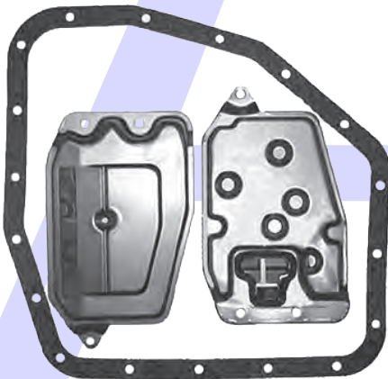
AISIN WARNER A245E, A246E, A247E Pan Gasket A245.GAS01 Filter A245.FIL01 1993-2002
