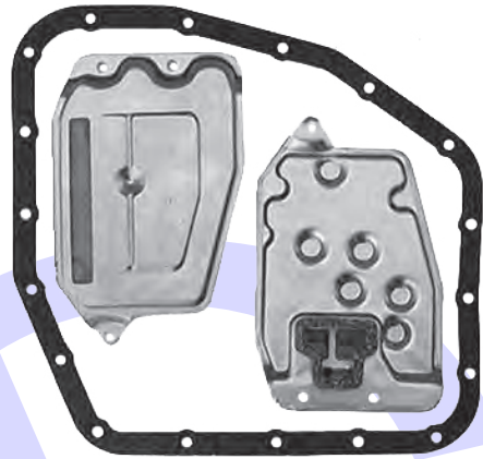
AISIN WARNER A245E Pan Gasket A245.GAS02 Filter A245.FIL02 2003-On
