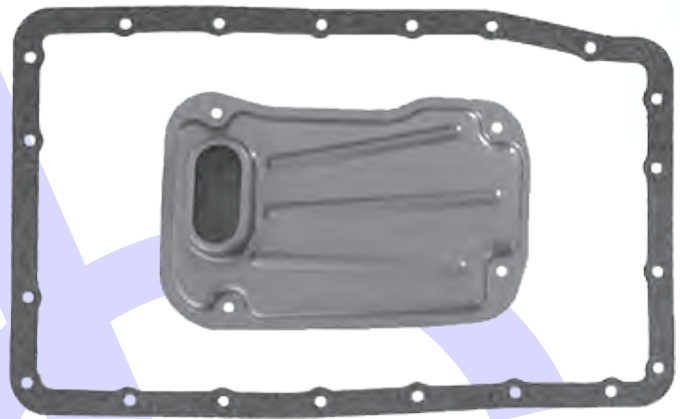
AISIN WARNER A750E 5 SPEED Pan Gasket A750.GAS01 Filter A750.FIL01 2003-ON
