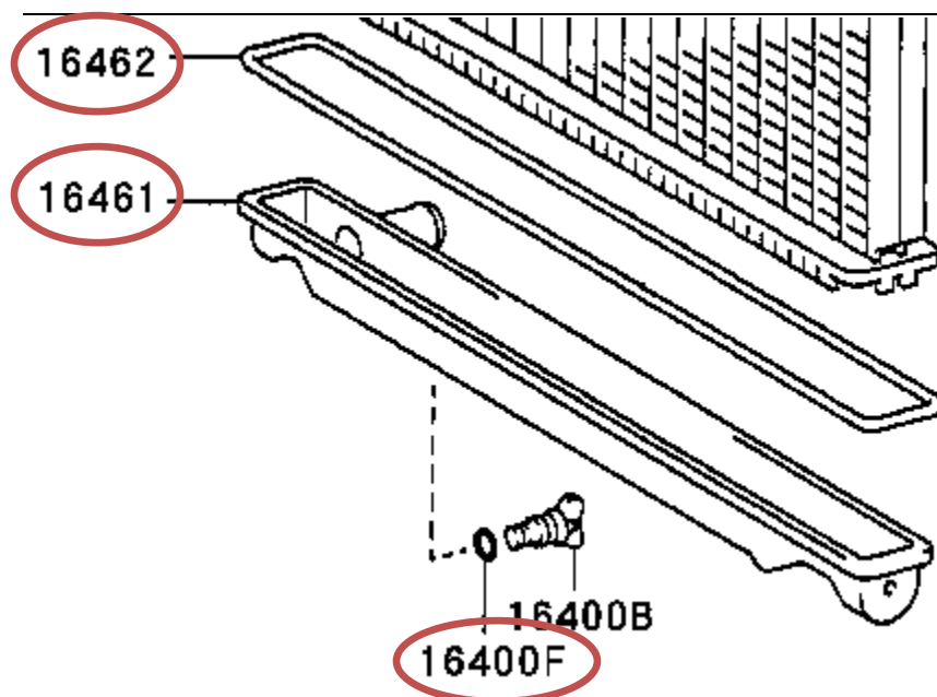
Tampa inferior do radiador (cód. 16461) + vedação (cód. 16462) + vedação (cód 16400F)
