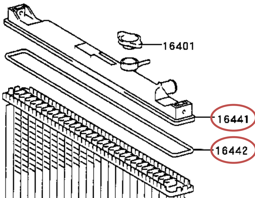
Tampa do radiador (cód. 16441) + vedação (cód. 16442)
