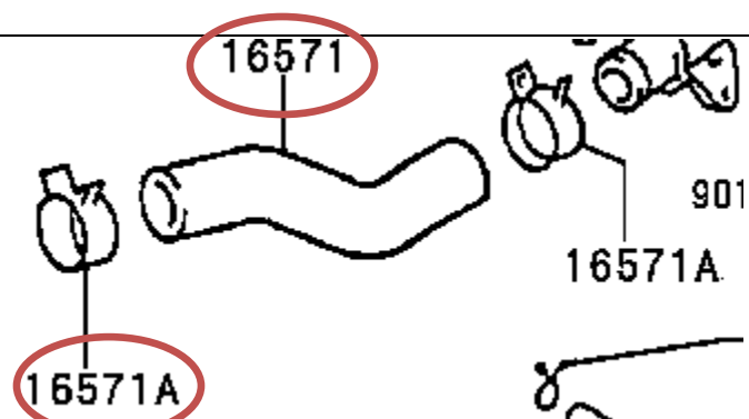
Mangueira do radiador superior (cód. 16571) + abraçadeira (cód 16571A)
