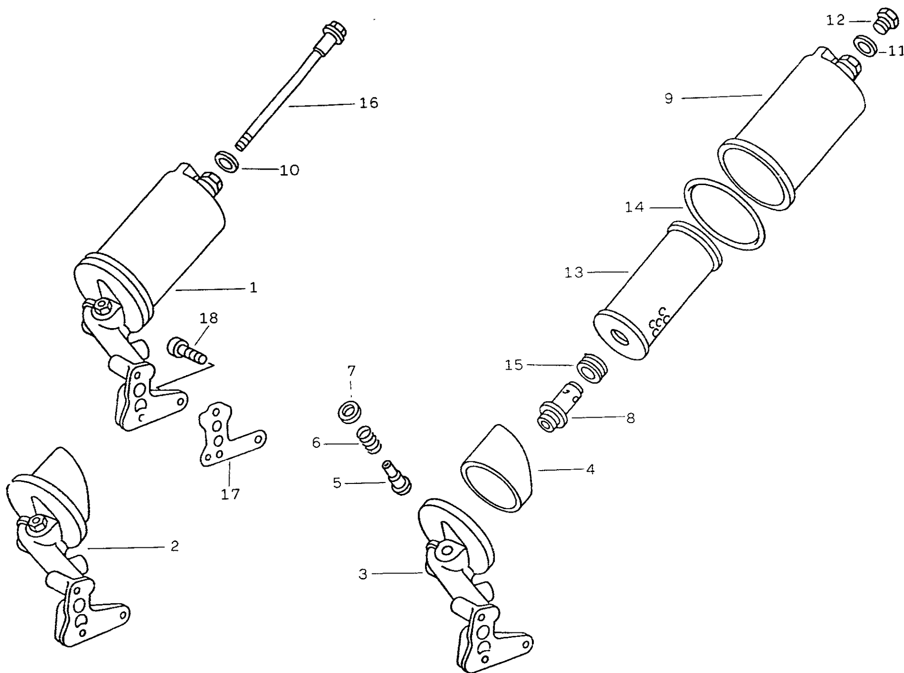
FIG. 11/20 - LUBRIFICAÇÃO DO MOTOR
