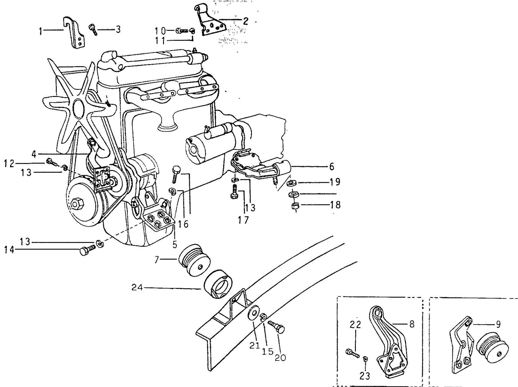
FIG. 10/23 - SUSPENSÃO DO MOTOR, TRANSMISSÃO E TRANSFERÊNCIA
