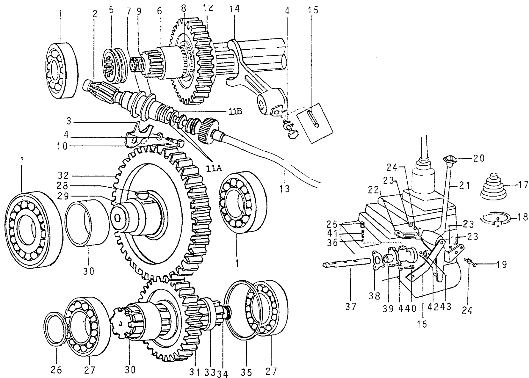
FIG. 02/04 - CAIXA DE TRANSFERÊNCIA - ENGRENAGENS
