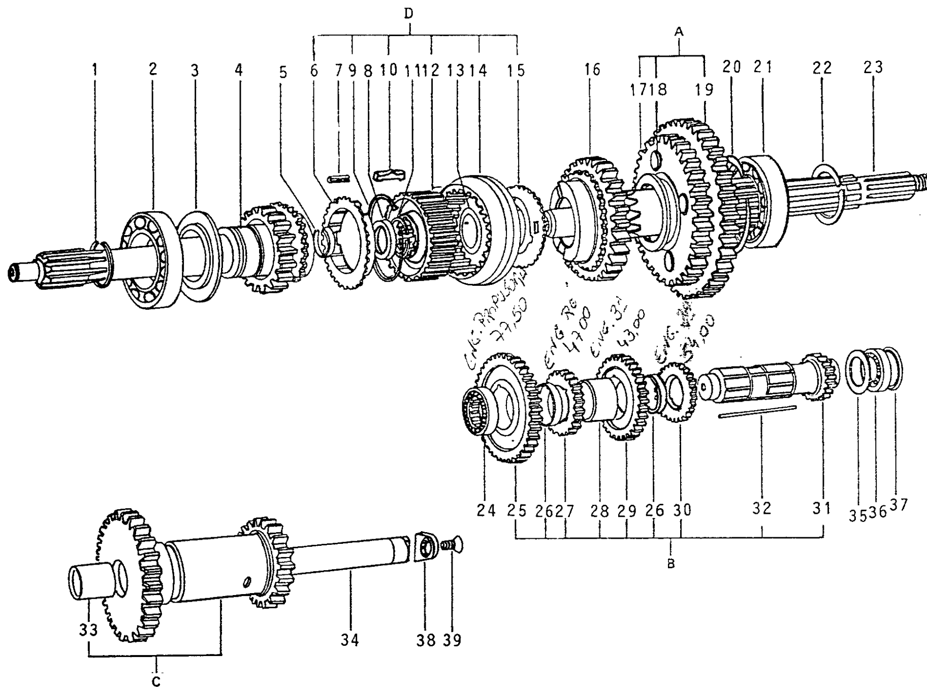
FIG. 02/02 - CAIXA DE MUDANÇAS - ENGRENAGENS
