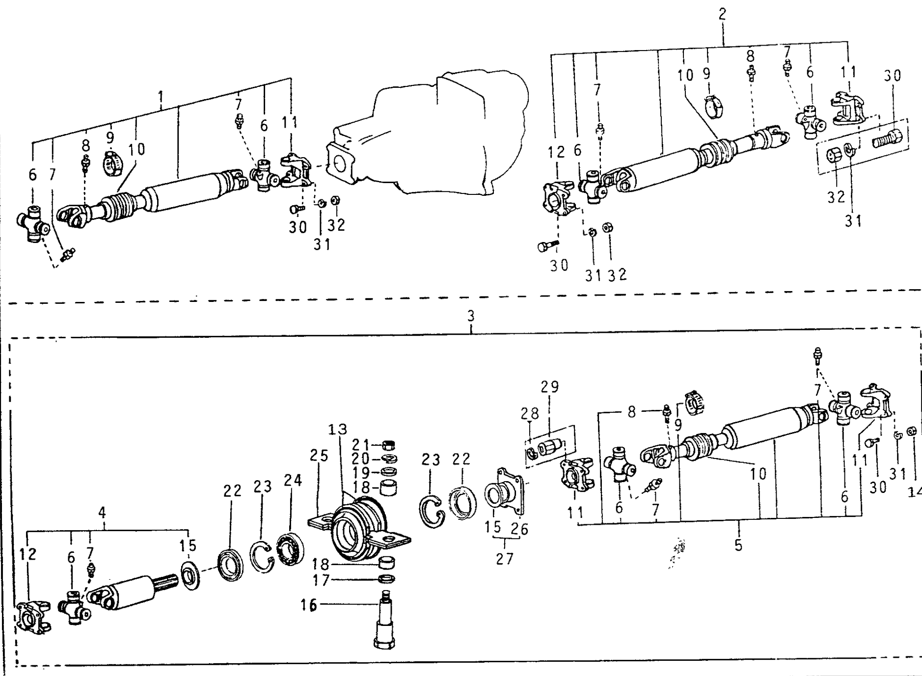
56 FIG. 02/11 - ÁRVORES DE TRANSMISSÃO
