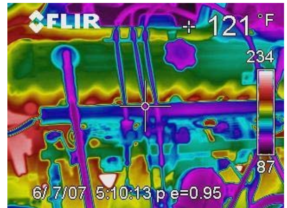
Motor
