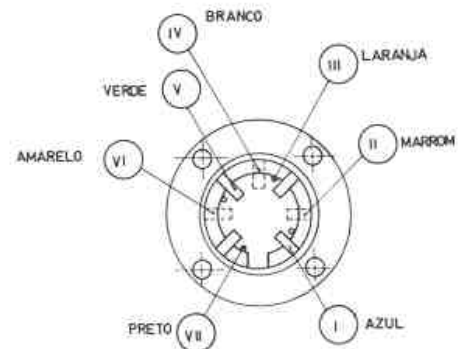
VISTA INTERNA DO PINO DA TOMADA DE FORÇA DO REBOQUE
