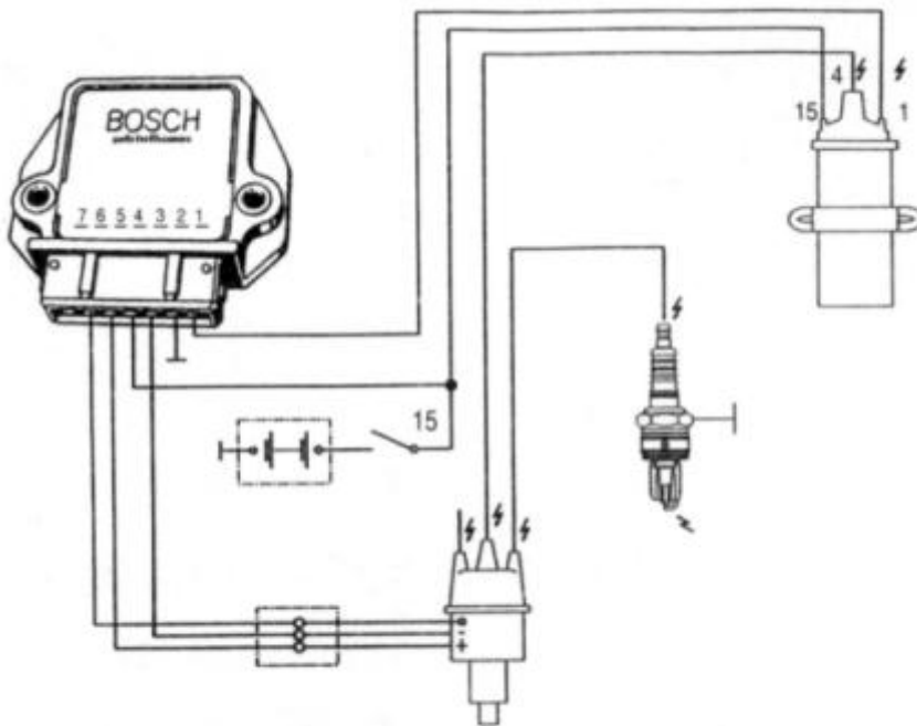
Sistema de ignição por efeito Hall- TZH (7 terminais)
