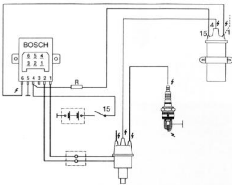
Sistema de ignição transistorizada TSZ-i (6 terminais)
