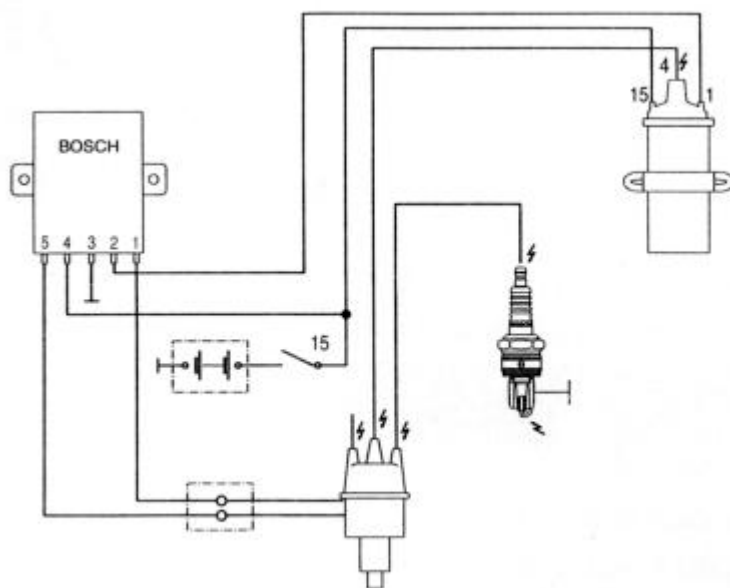
Sistema de ignição mini (5 terminais)
