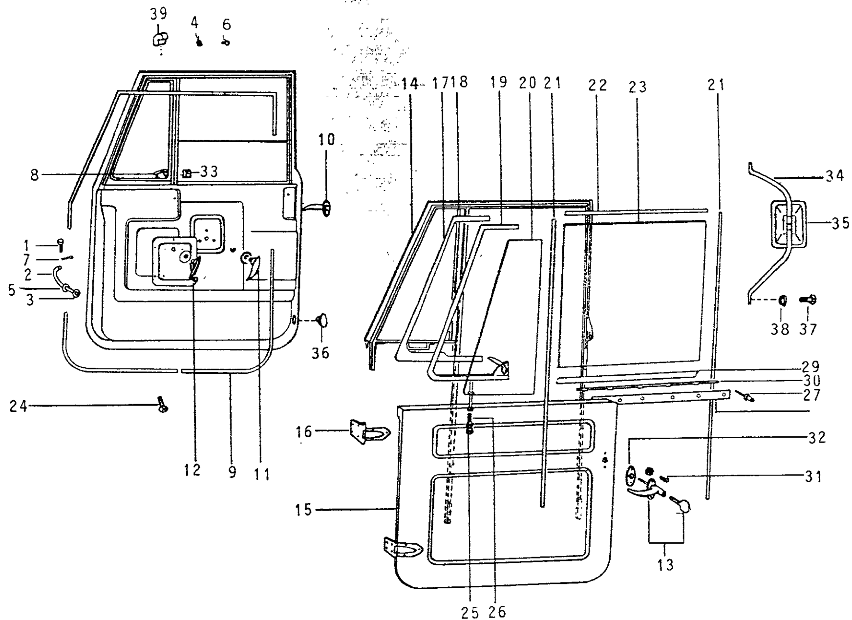
FIG. 08/11 - PORTAS DIANTEIRAS
