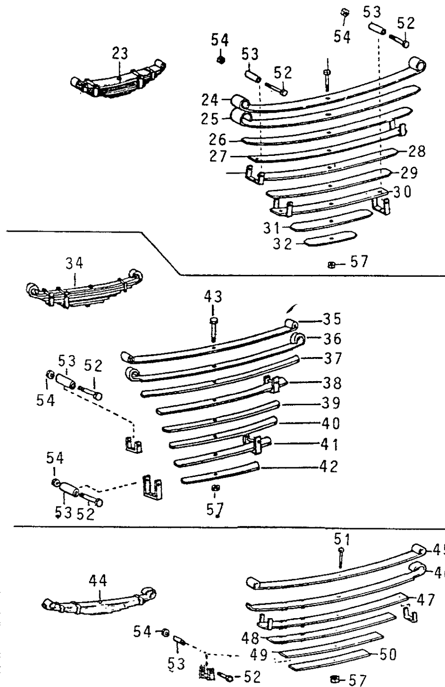
FIG. 06/03 - SUSPENSÃO TRASEIRA (PICK-UPS, CABINE DUPLA)
