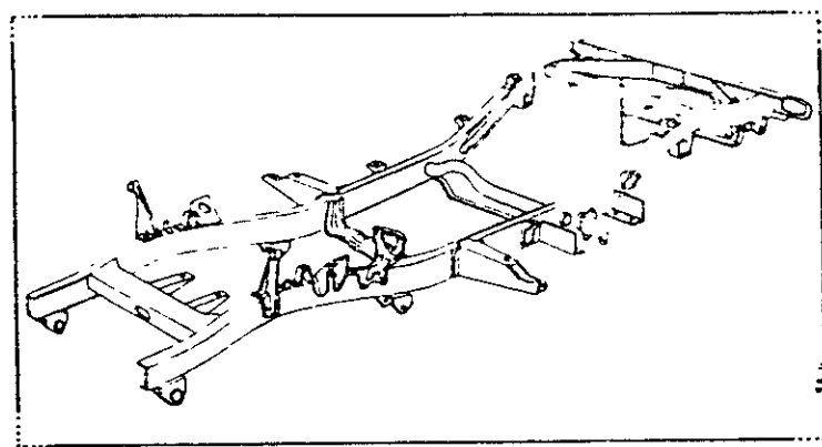
FIG. 07/01 - CHASSI P/ LONA, AÇO, PERUA E COMPONENTES
