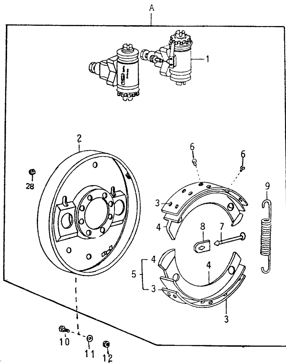
135 FIG. 05/07 - FREIO DA RODA - CILINDROS E PRATOS
