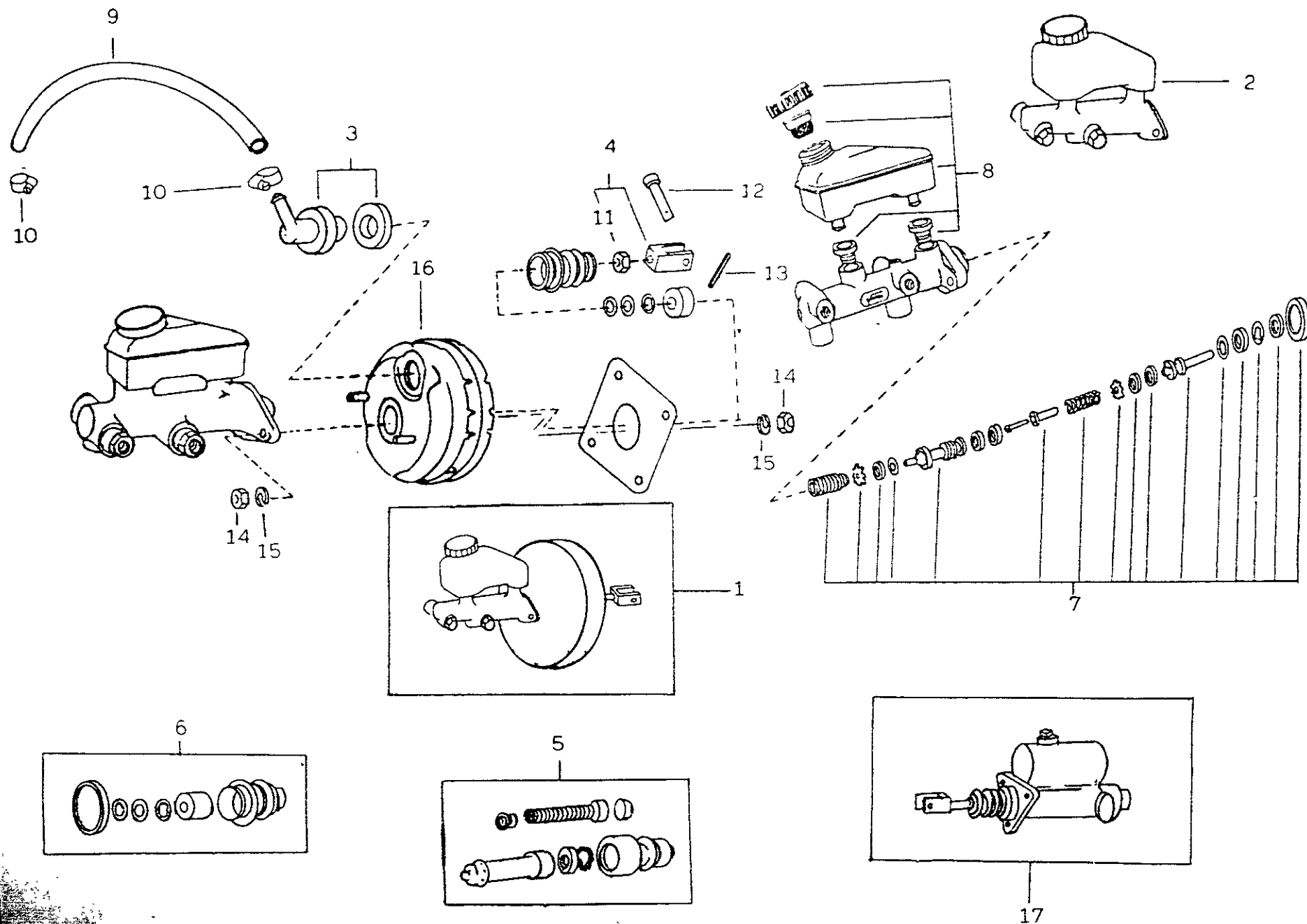
FIG. 05/04 - SERVO FREIO (ANTIGO)
