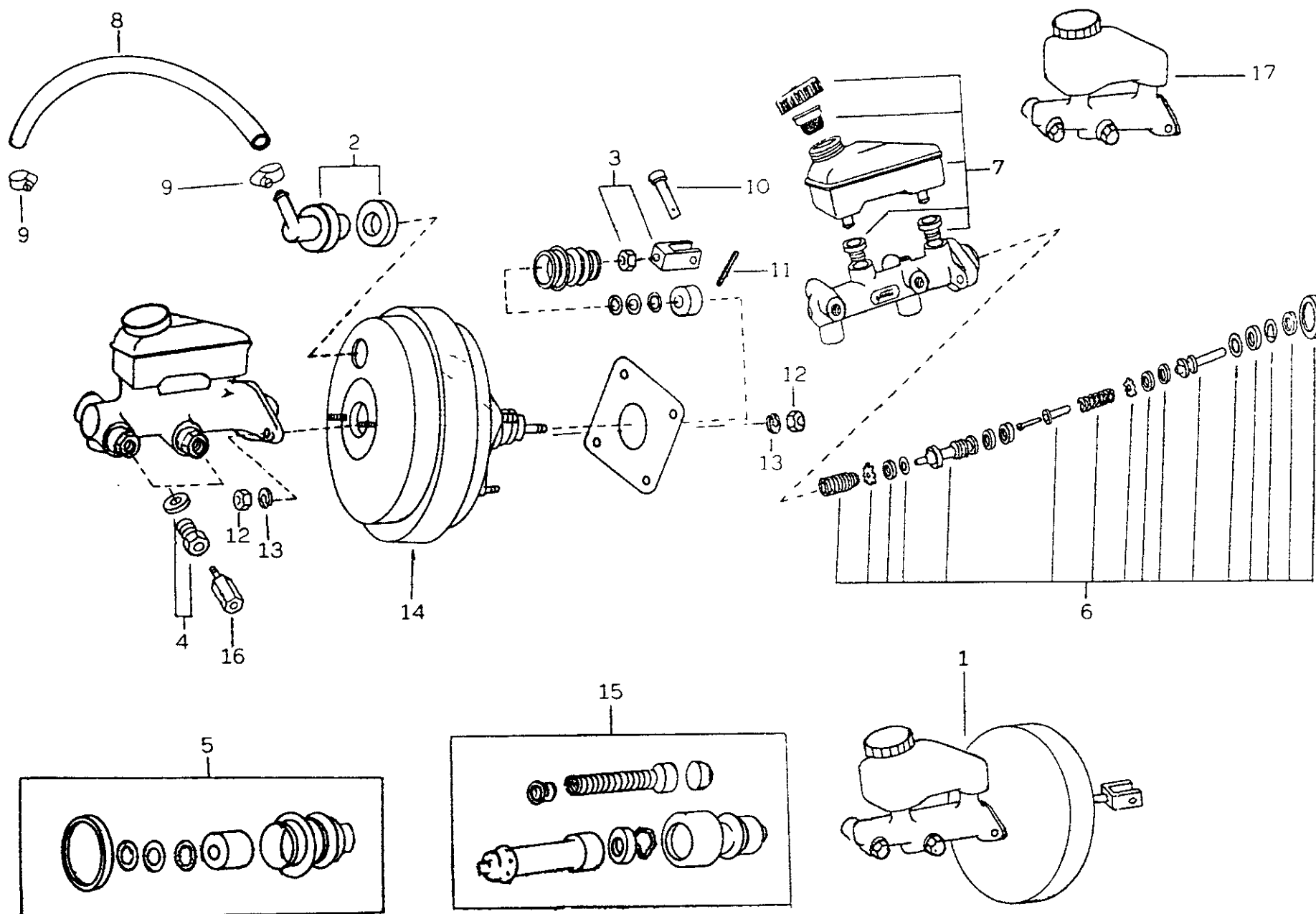
FIG. 05/04A - SERVÔ FREIO (ATUAL)
