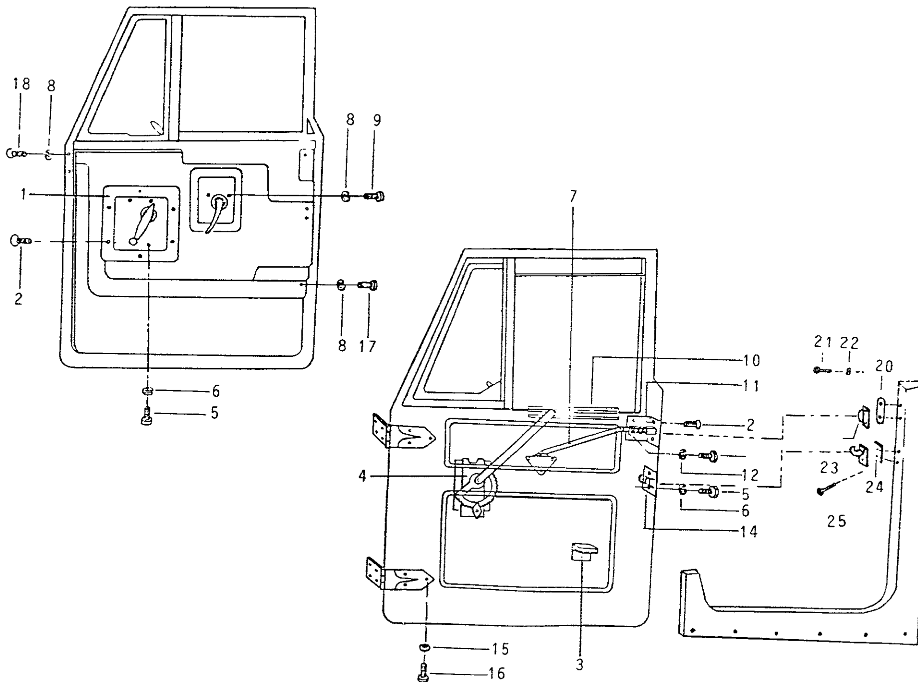
FIG. 08/12 - PORIAS (COMPONENTES)
