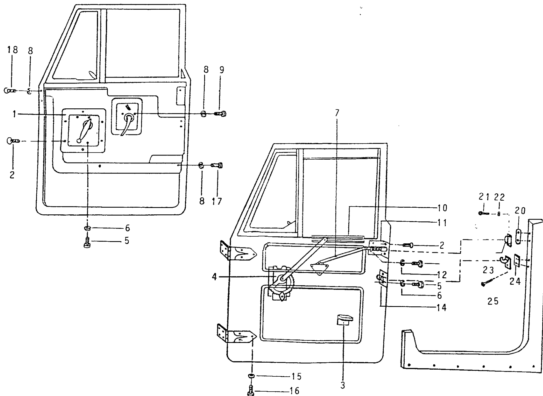
FIG. 08/12 - PORTAS (COMPONENTES)
