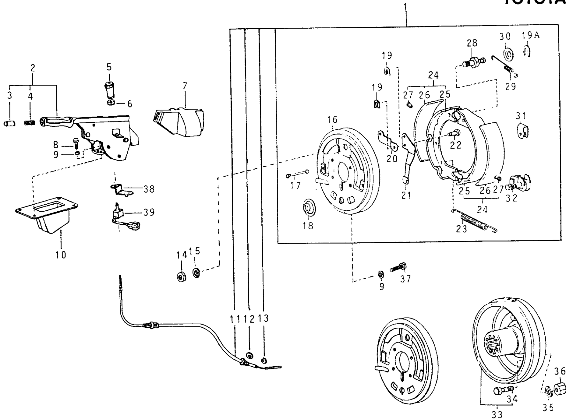
FIG. 05/02 - FREIO DE ESTACIONAMENTO
