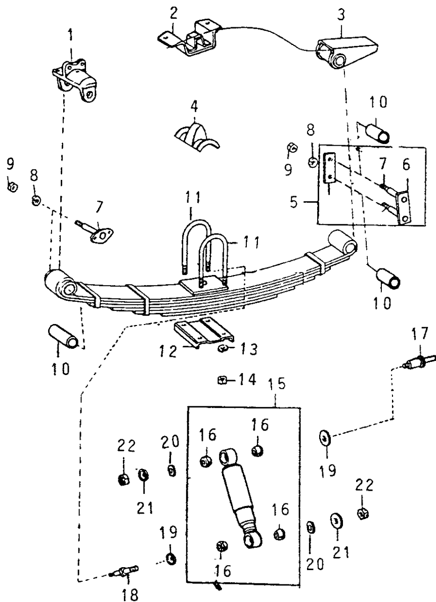
FIG. 06/02 - SUSPENSÃO TRASEIRA (LONA, AÇO, PERUA)
