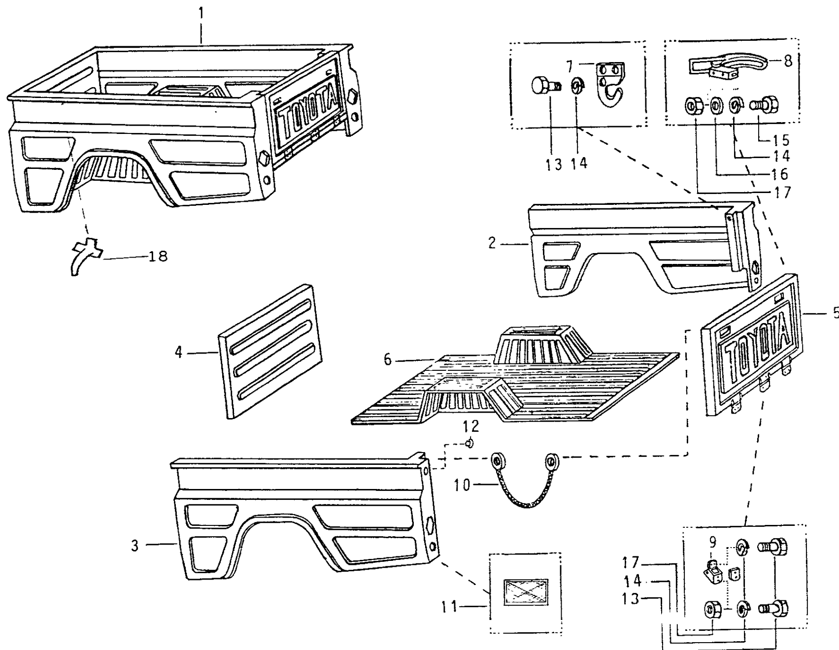
FIG. 08/06 - CAÇAMBA PICK-UPS E CABINE DUPLA
