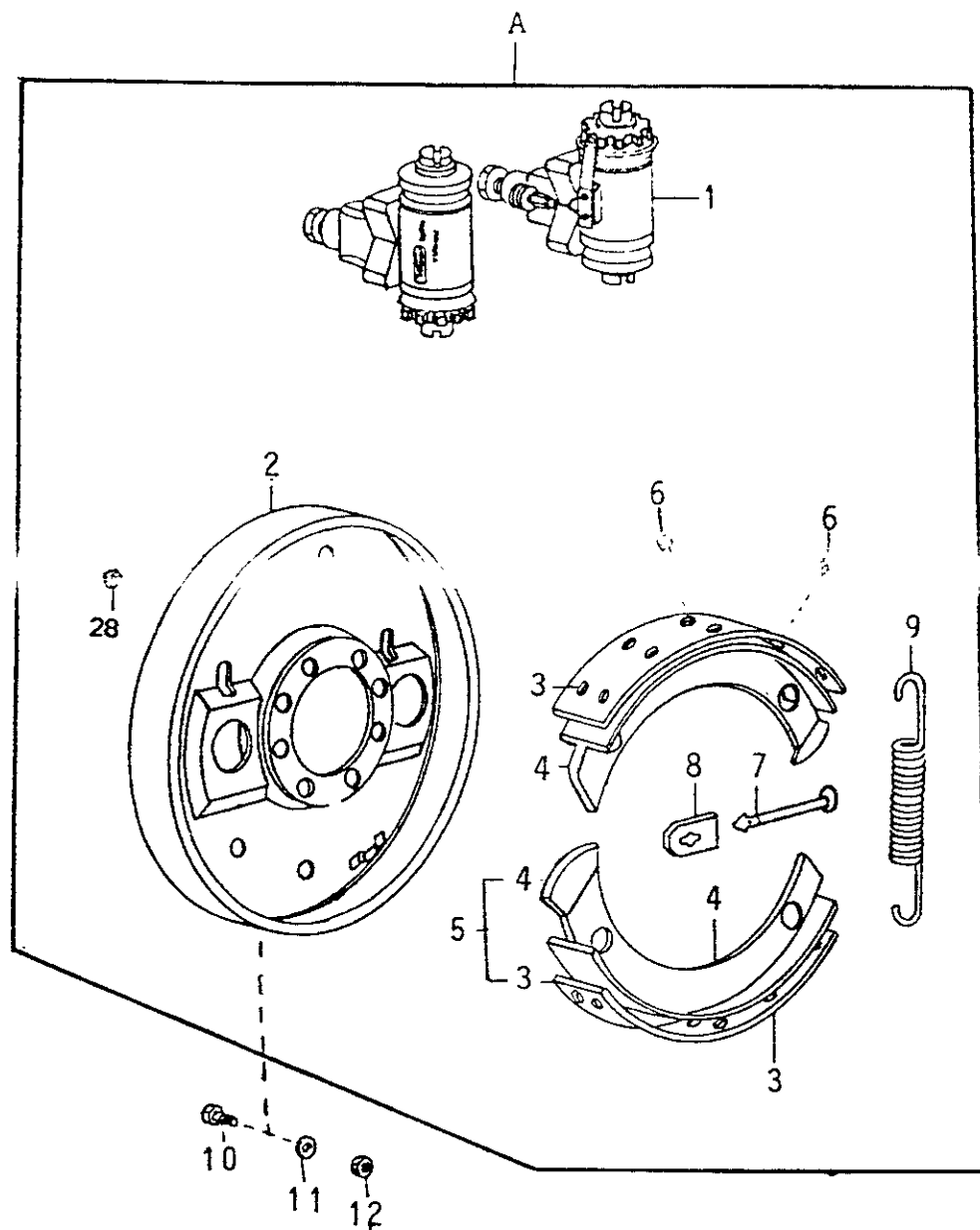
FIG. 05/07 - FREIO DA RODA - CILINDROS E PRATOS
