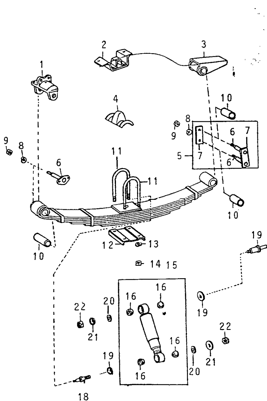
FIG. 06/03 - SUSPENSÃO TRASEIRA (PICK-UPS, CABINE DUPLA)
