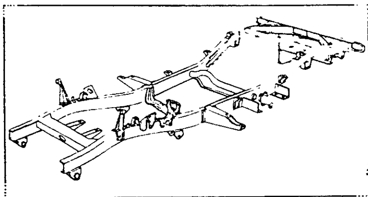
FIG. 07/01 - CHASSI P/ LONA, AÇO, PERUA E COMPONENTES
