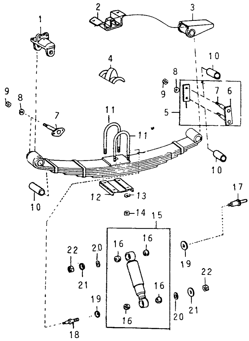
FIG. 06/02 - SUSPENSÃO TRASEIRA (LONA, AÇO, PERUA)
