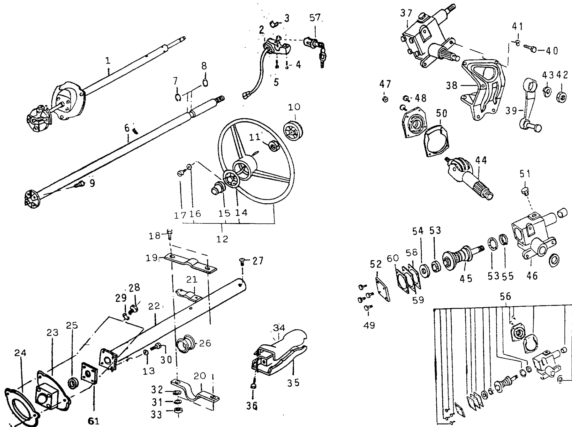
36 FIG. 04/02 - SISTEMA DE DIREÇÃO - CAIXA, COLUNA E VOLANTE
