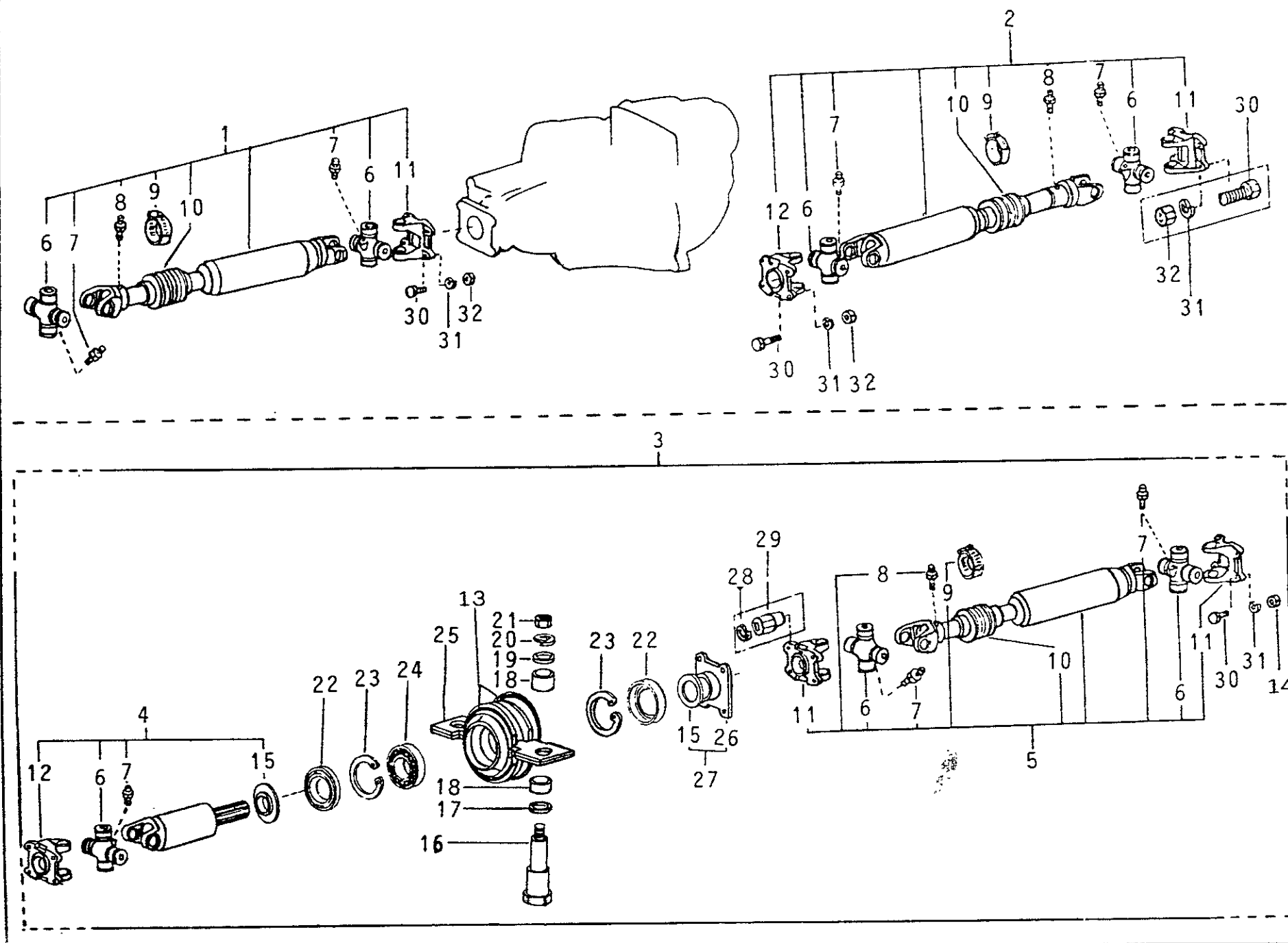
FIG. 02/11 - ÁRVORES DE TRANSMISSÃO
