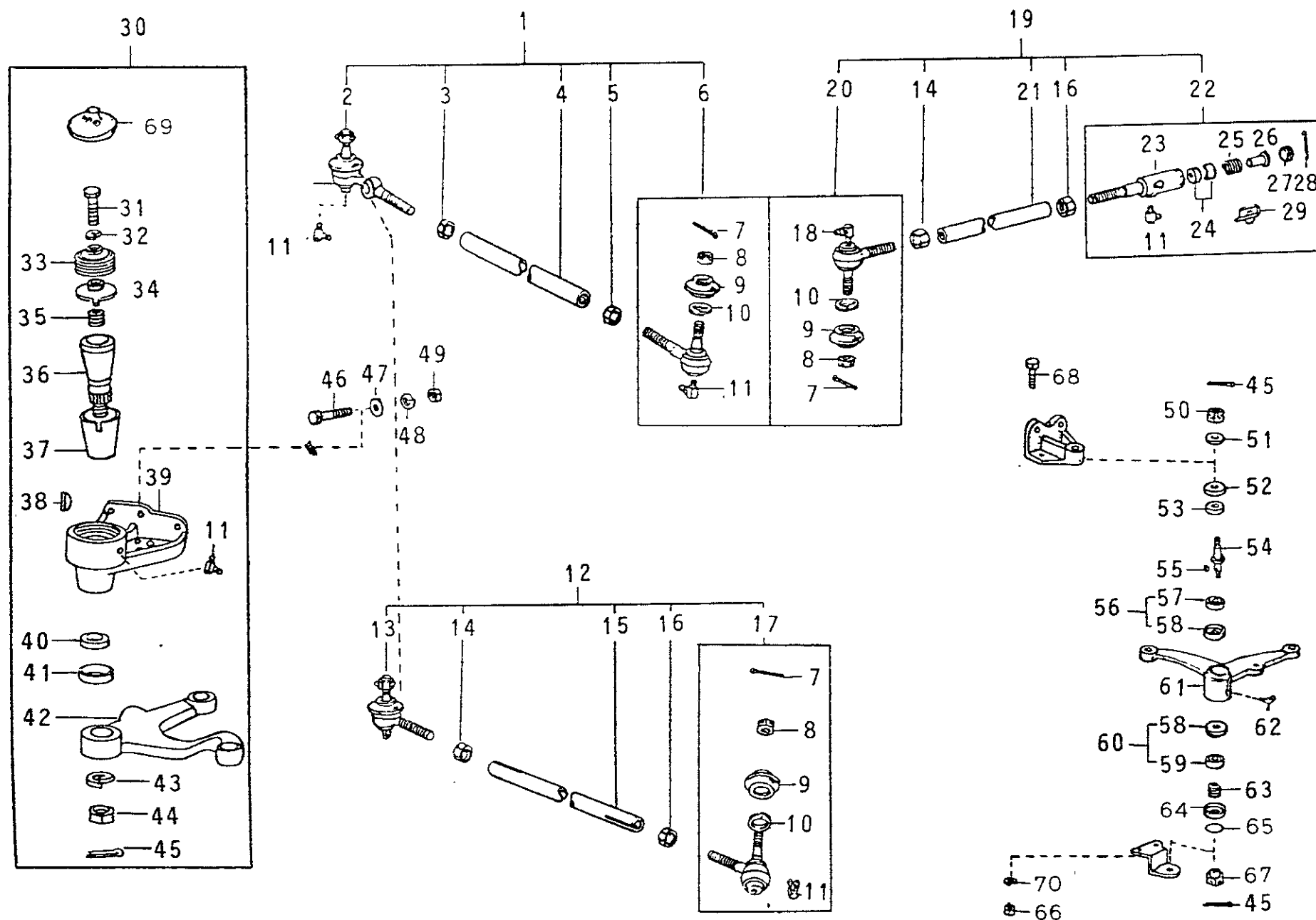
FIG. 04/03 - SISTEMA DE DIREÇÃO - BARRAS DE LIGAÇÃO
