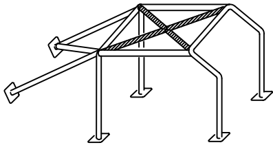
Dessin / Drawing N° 253-9A
