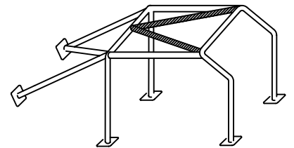
Dessin / Drawing N° 253-9C
