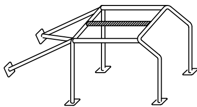
Dessin / Drawing N° 253-9D
