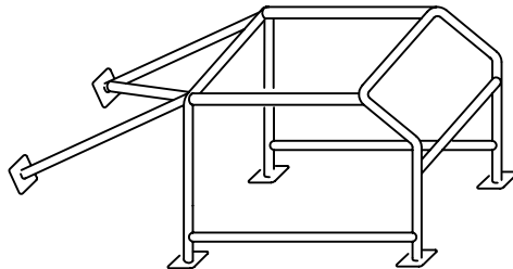
Dessin / Drawing N°283-6
