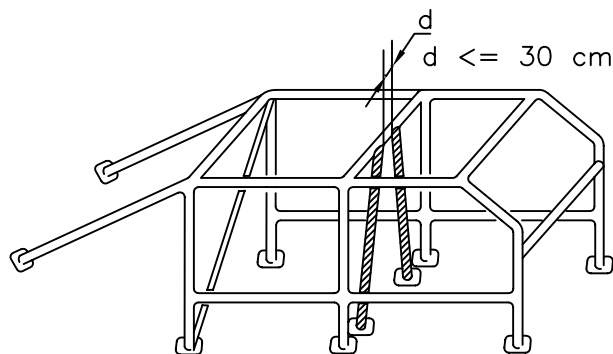
Dessin / Drawing N°283-5
